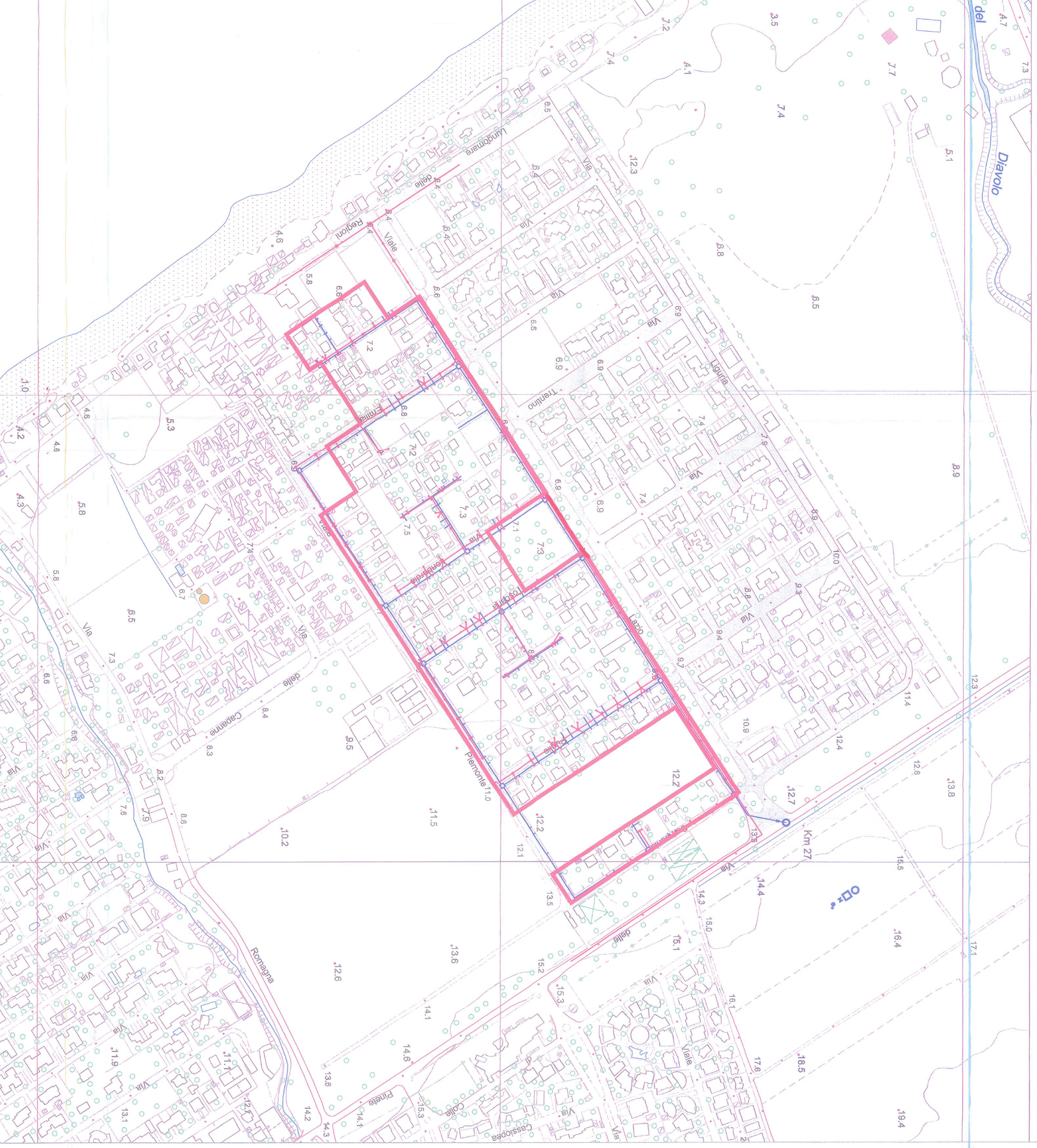
TRACCIATO IMPIANTO FOGNARIO ED IDRICO - STATO DI FATTO - rapp. 1:2000
