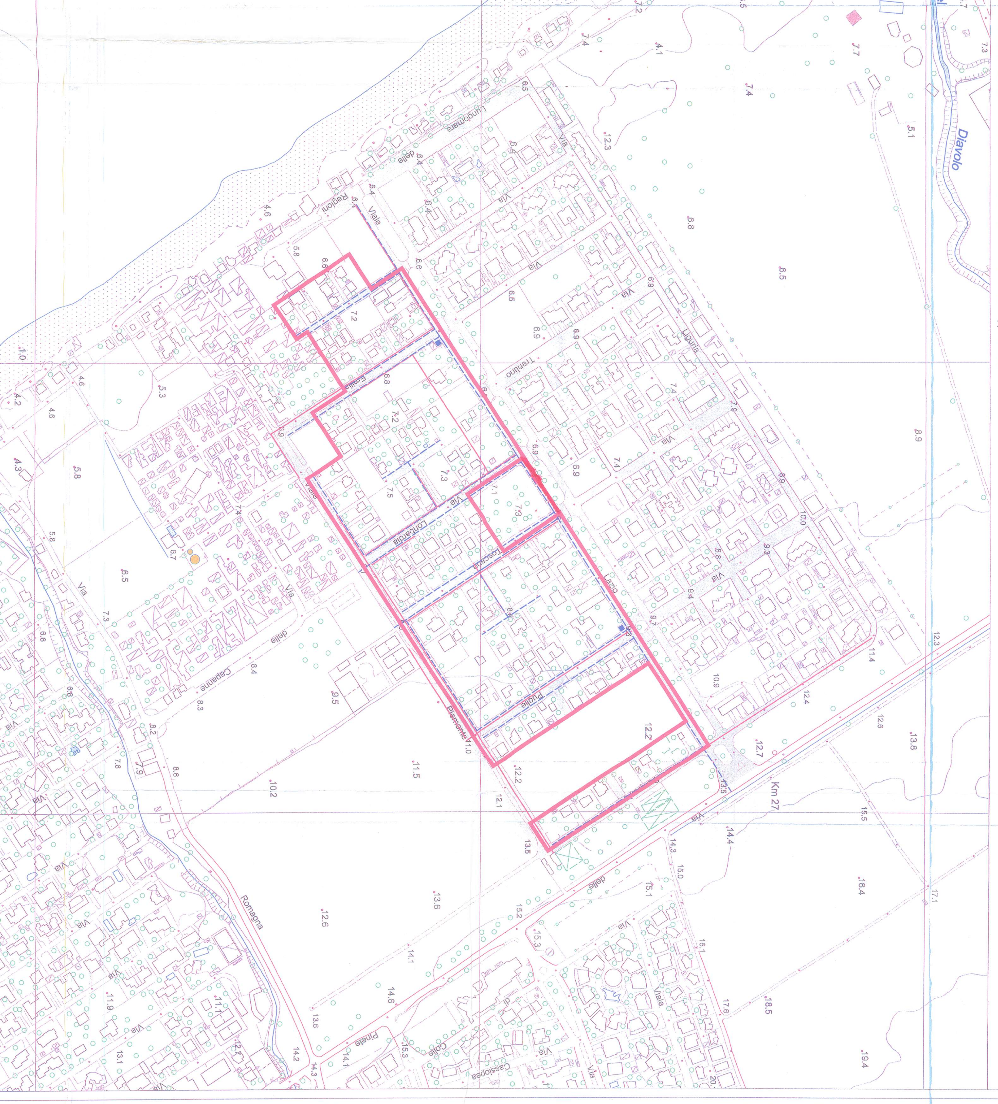
TRACCIATO LINEA ELETTRICA E TELEFONICA - STATO DI FATTO - rapp. 1:2000
