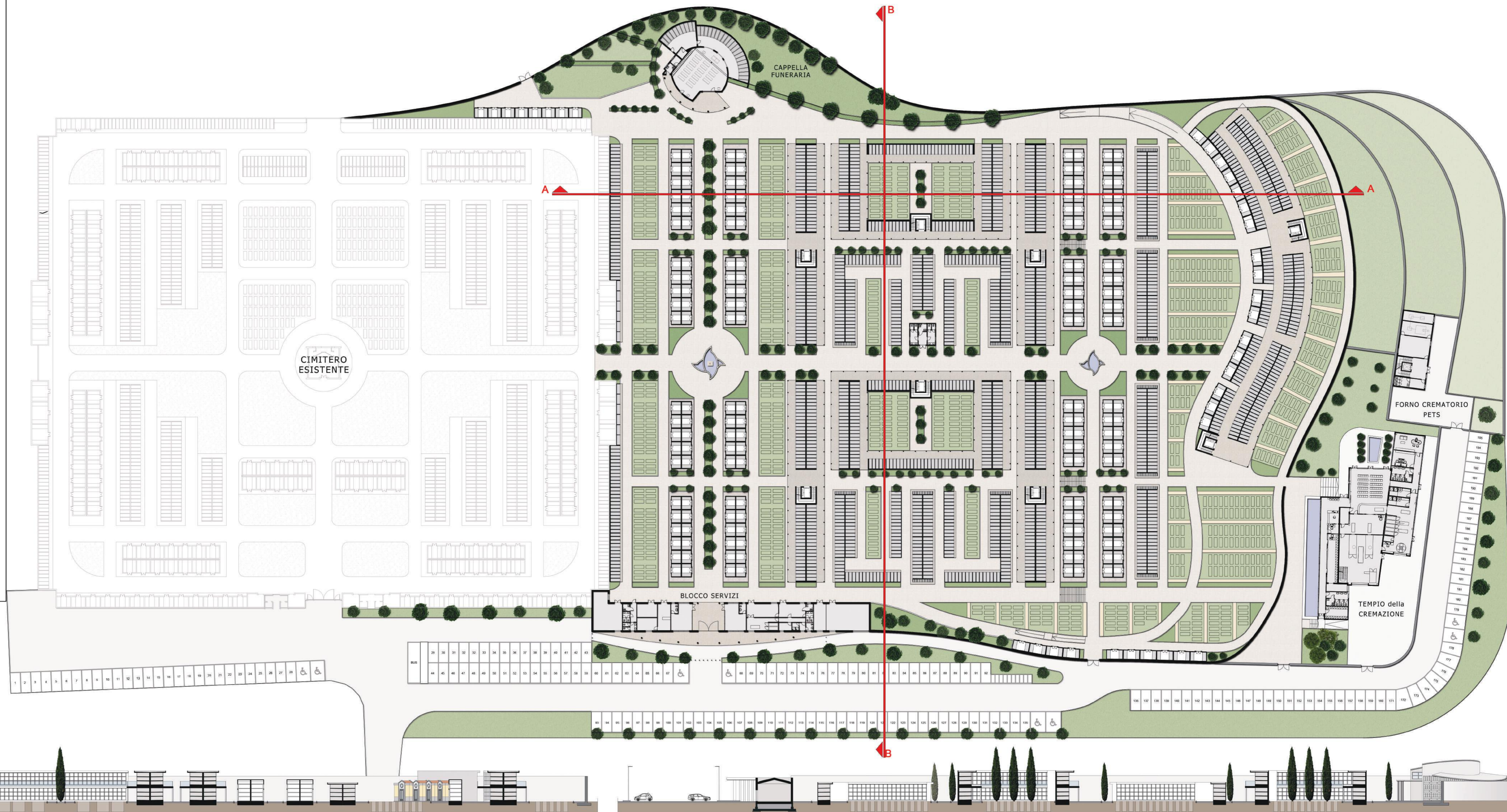
PROFILO BB
